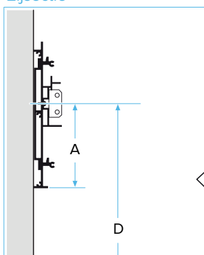
Bovenaanzicht
